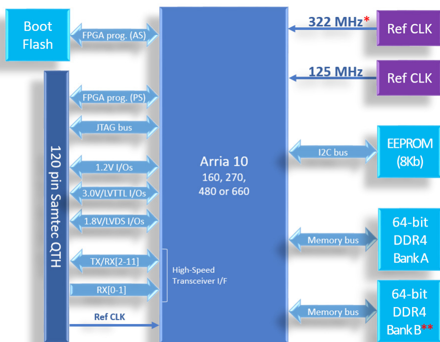
FDB Block Diagram
