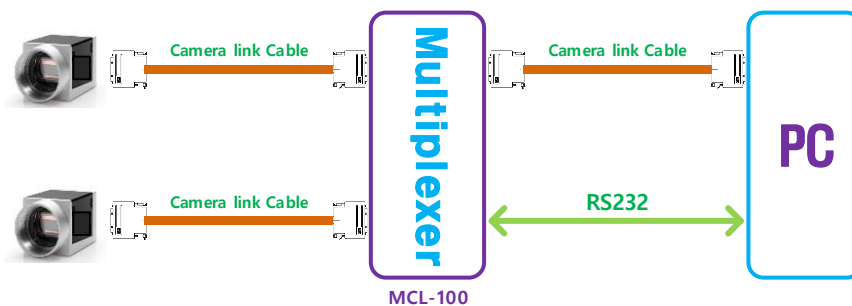
<표준 설치도>
