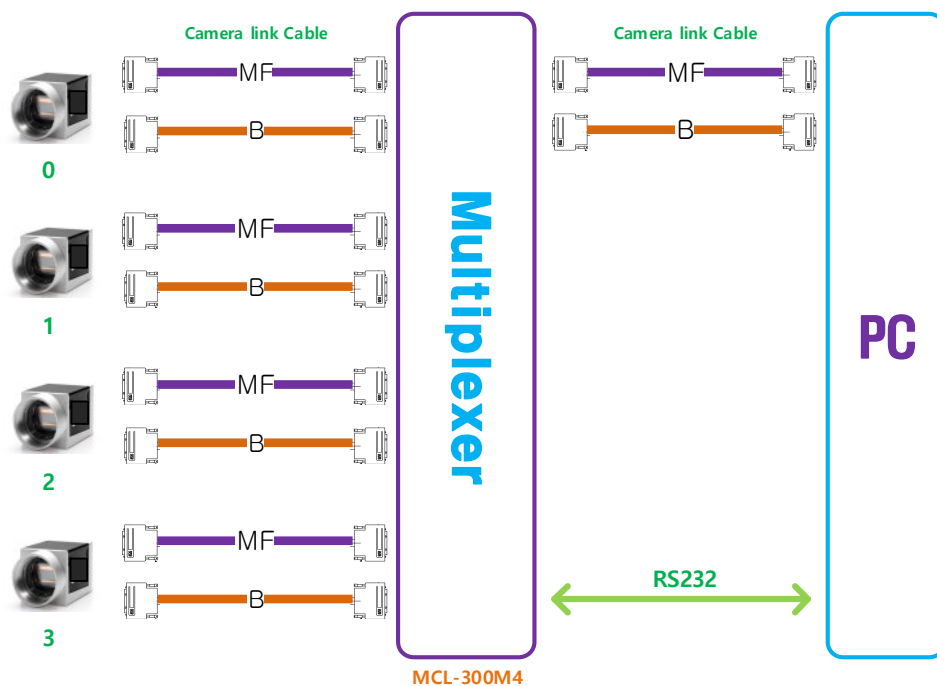
〈표준 설치도〉
