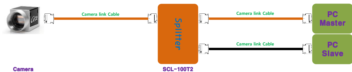
〈표준 설치도〉
