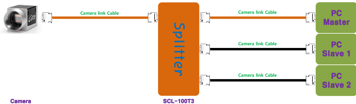
<표준 설치도>
