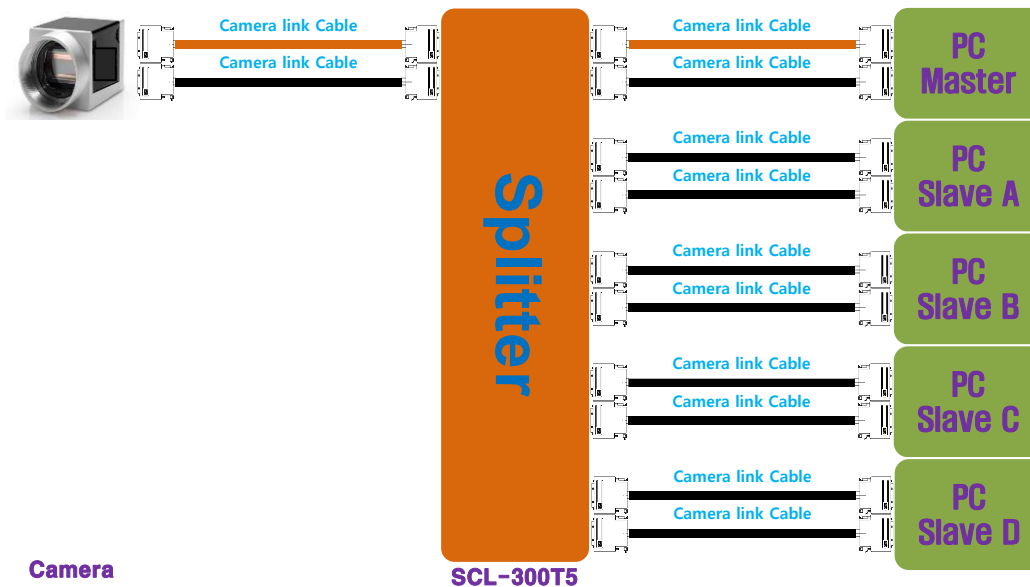
<표준 설치도>
